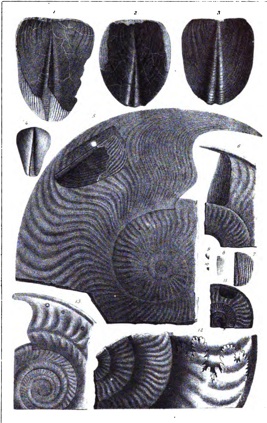
Quenstedt, Jura.
